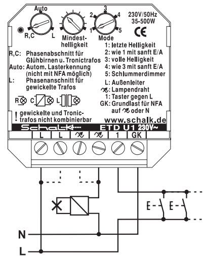
Anschluss mit Netz-Feld-Abschaltautomat und Tronictrafo
