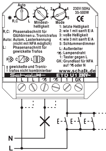
Anschluss ohne Netz-Feld-Abschaltautomat
