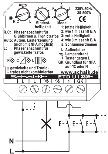
Anschluss mit Netz-Feld-Abschaltautomat
