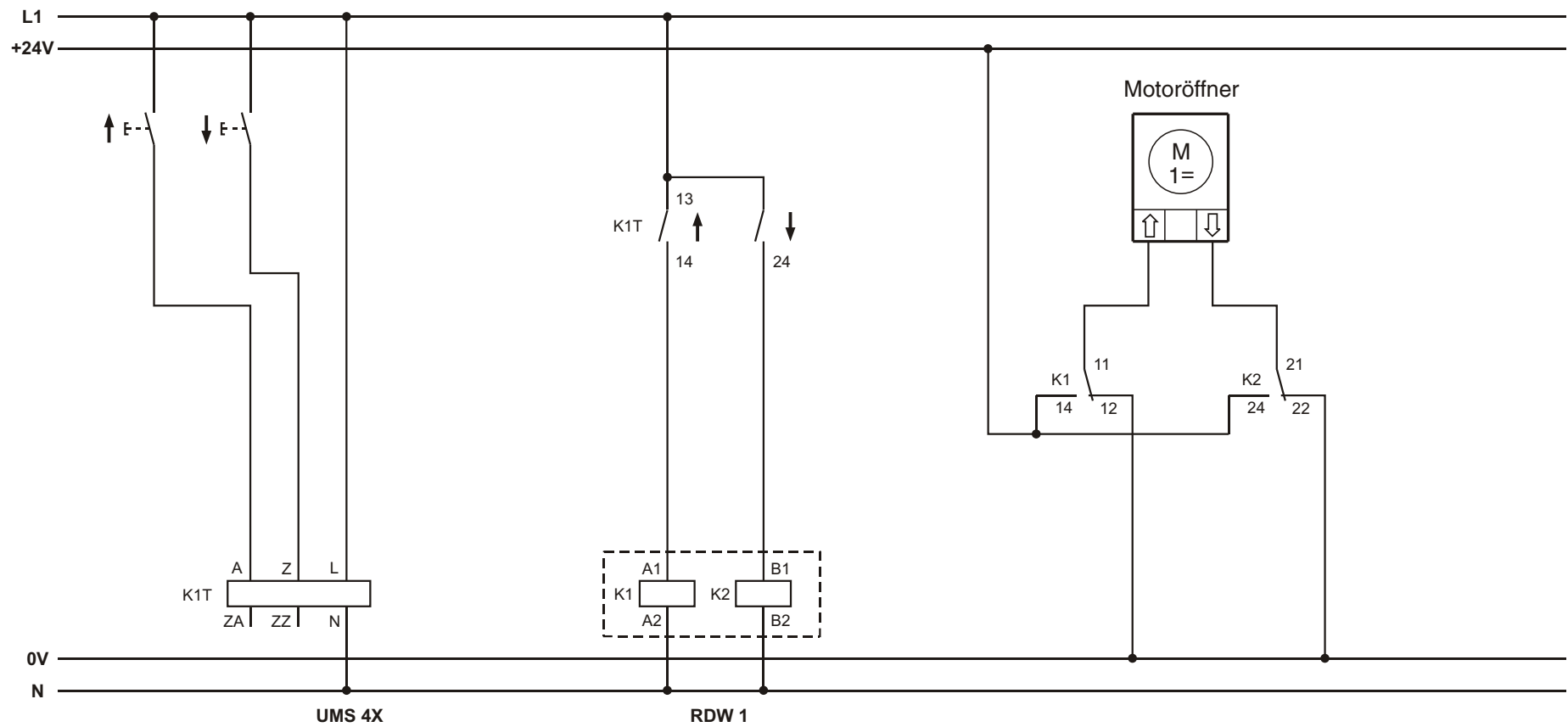
Anschlussbeispiel RDW 1
