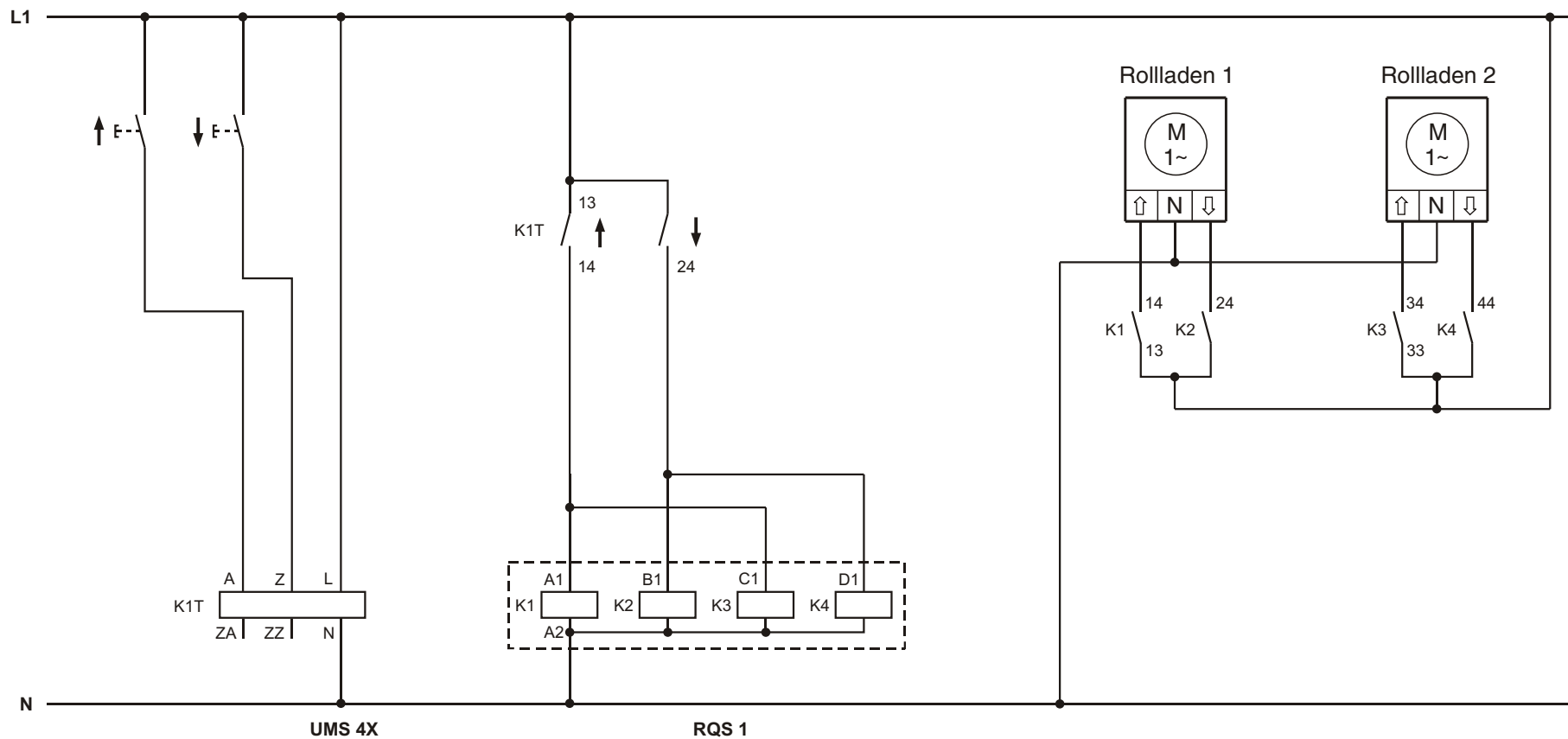
Anschlussbeispiel RQS 1
